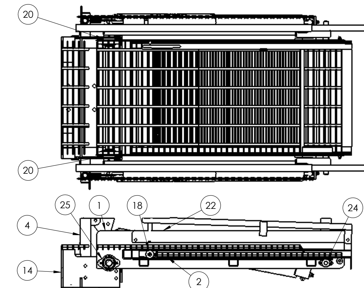
SECTION A-A
